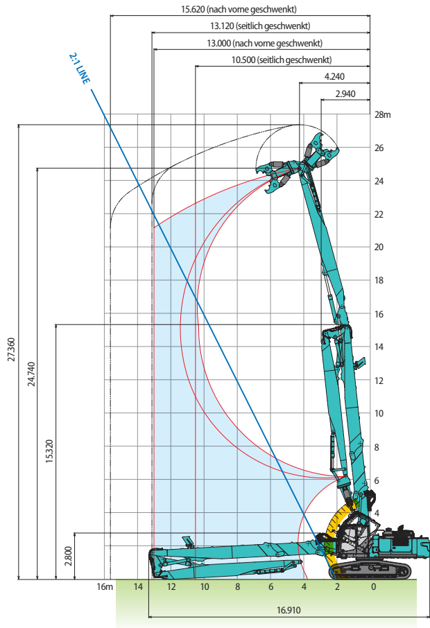
SK400D LC 8,7 m Stiel + 2,4 m Zwischenausleger Max. Werkzeuggewicht = 2.600 kg
