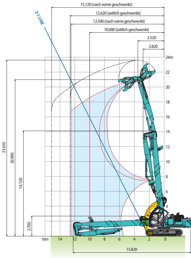
SK350D LC 6,1 m Stiel Max. Werkzeuggewicht = 2.600 kg
