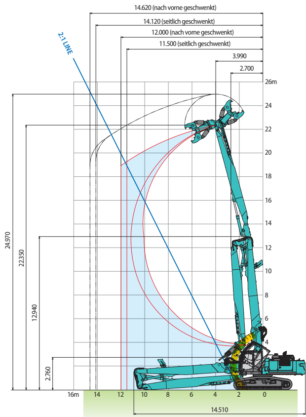
SK400D LC 8,7 m Stiel Max. Werkzeuggewicht = 2.600 kg
